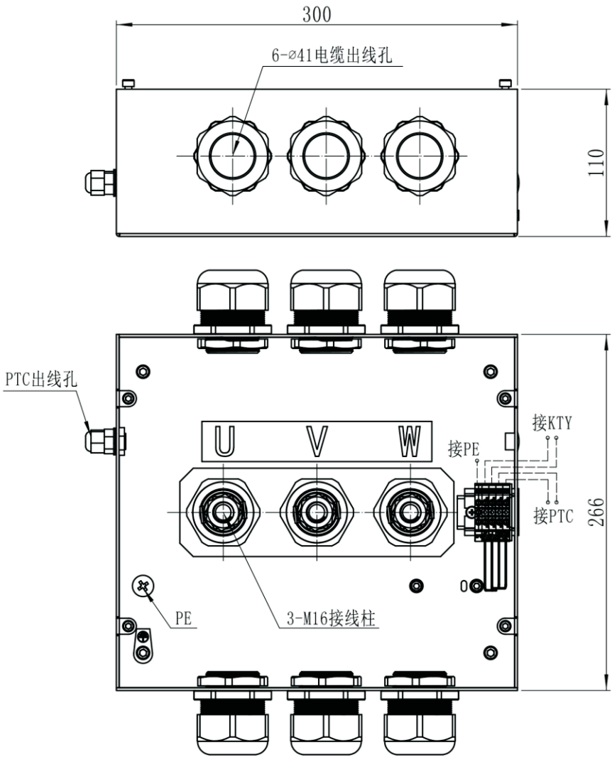
SMM460油冷接线图
