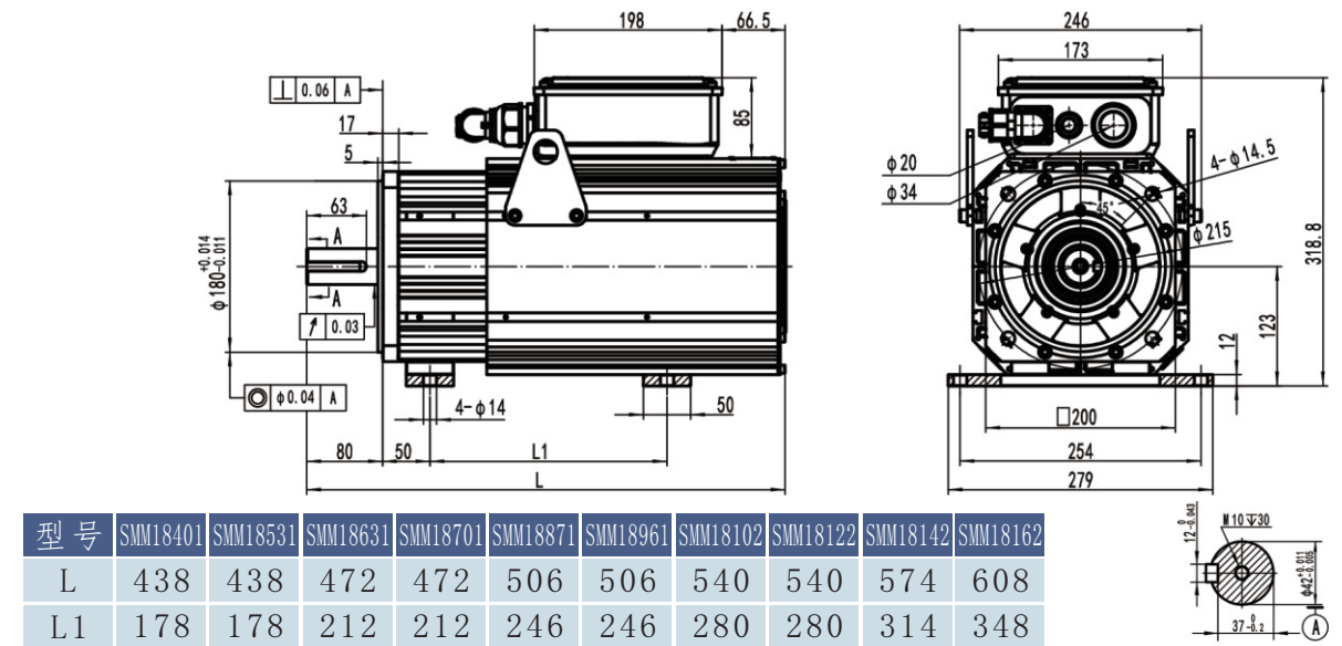
SMM180-H5系列风冷卧式电机外形尺寸图&amp;性能参数一览表
