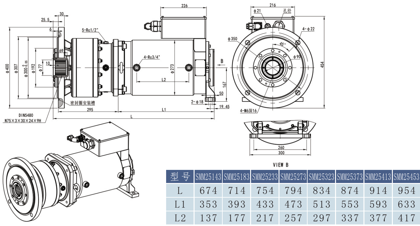
SMM250系列带减速箱电机外形尺寸&性能数一览表
