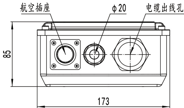
SMM18风冷接线图
