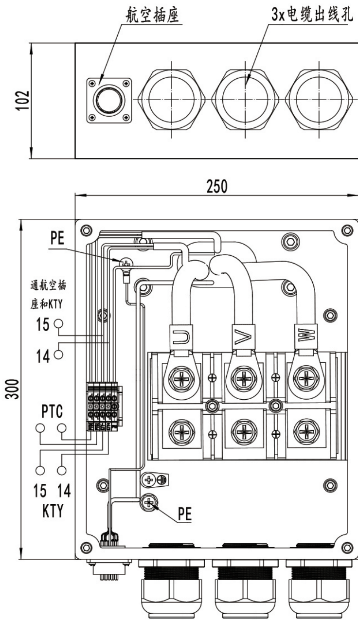
SMM30油冷接线图
