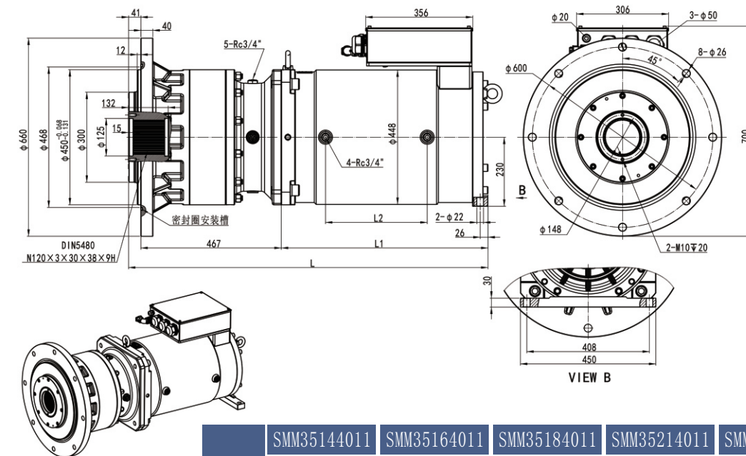
SMM350系列带减速箱电机外形尺寸&性能数一览表
