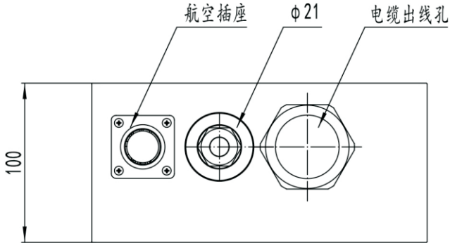
SMM25油冷接线图
