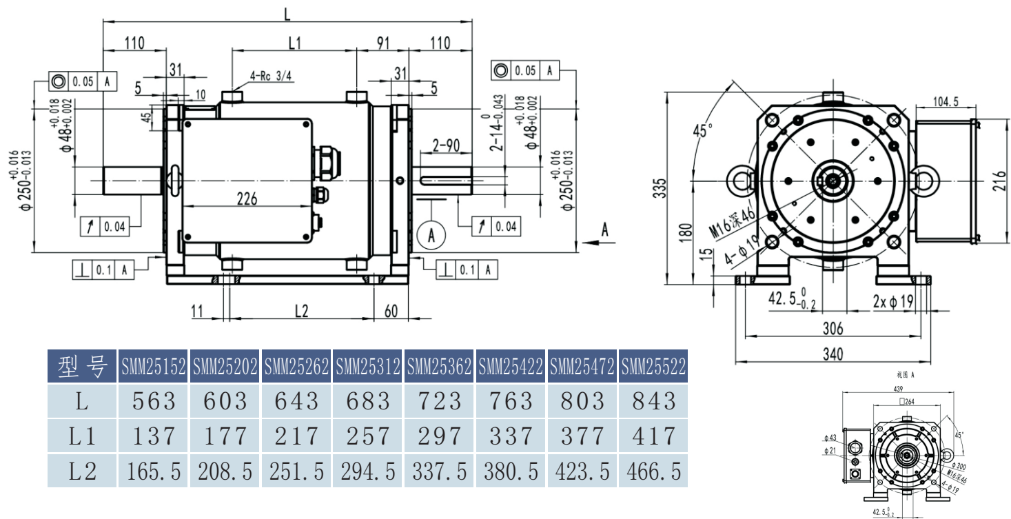
SMM250油冷平键双出轴电机外形尺寸图&性能参数一览表
