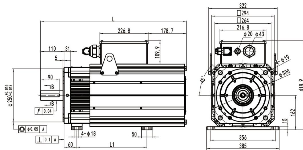
SMM250系列风冷卧式电机外形尺寸图&性能参数一览表
