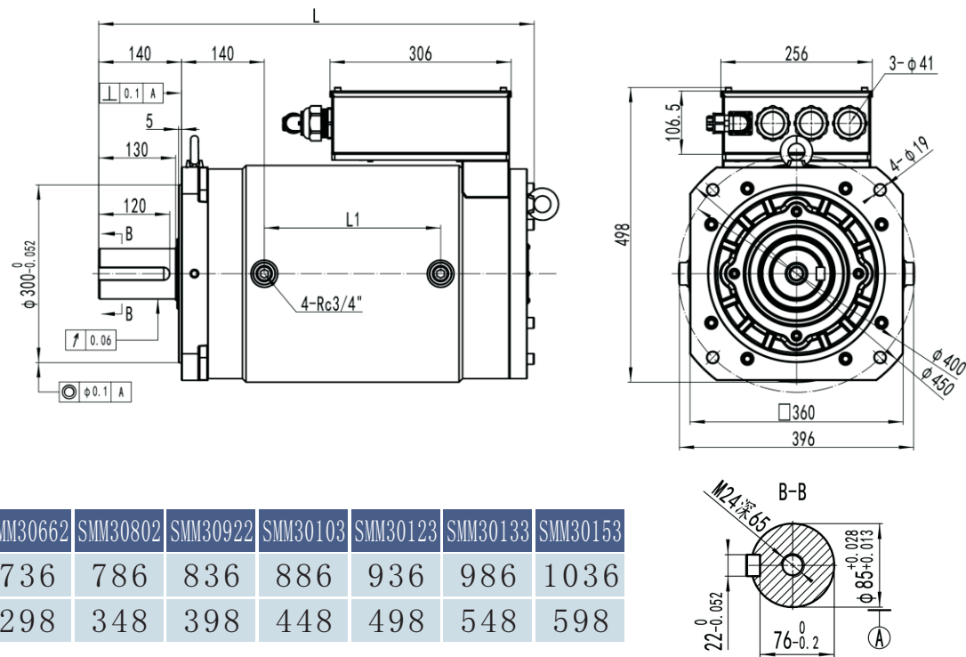
SMM300系列油冷立式电机外形尺寸图&性能参数一览表
