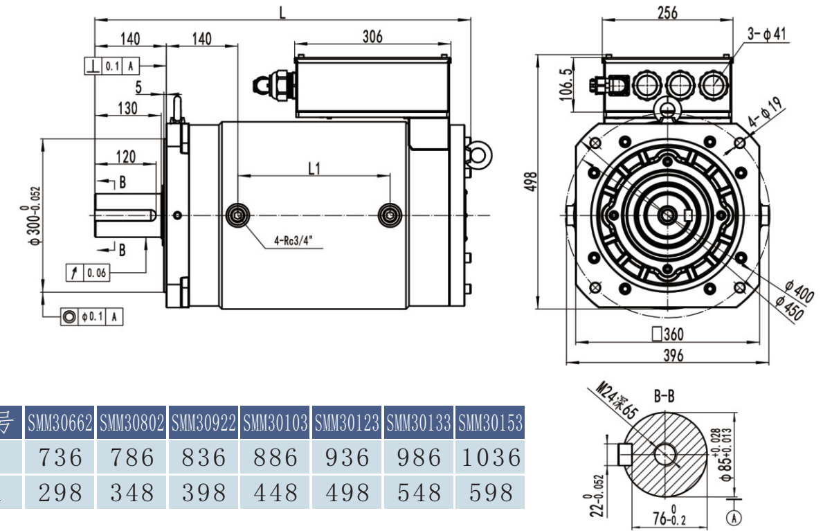
SMM300系列油冷立式熔胶电机外形尺寸图&amp;性能参数一览表
