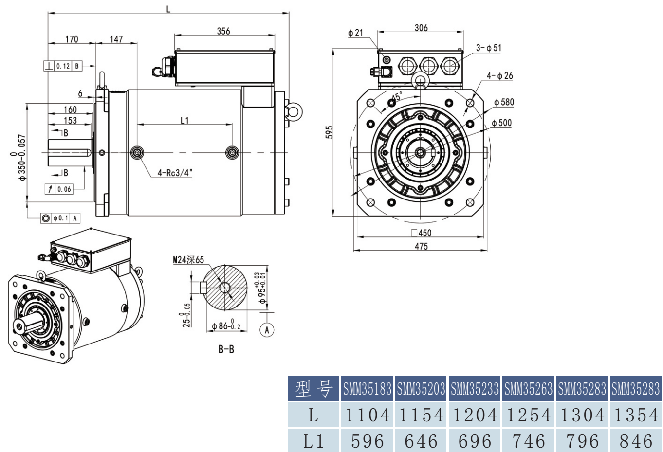
SMM350系列油冷电机外形尺寸&性能数一览表1
