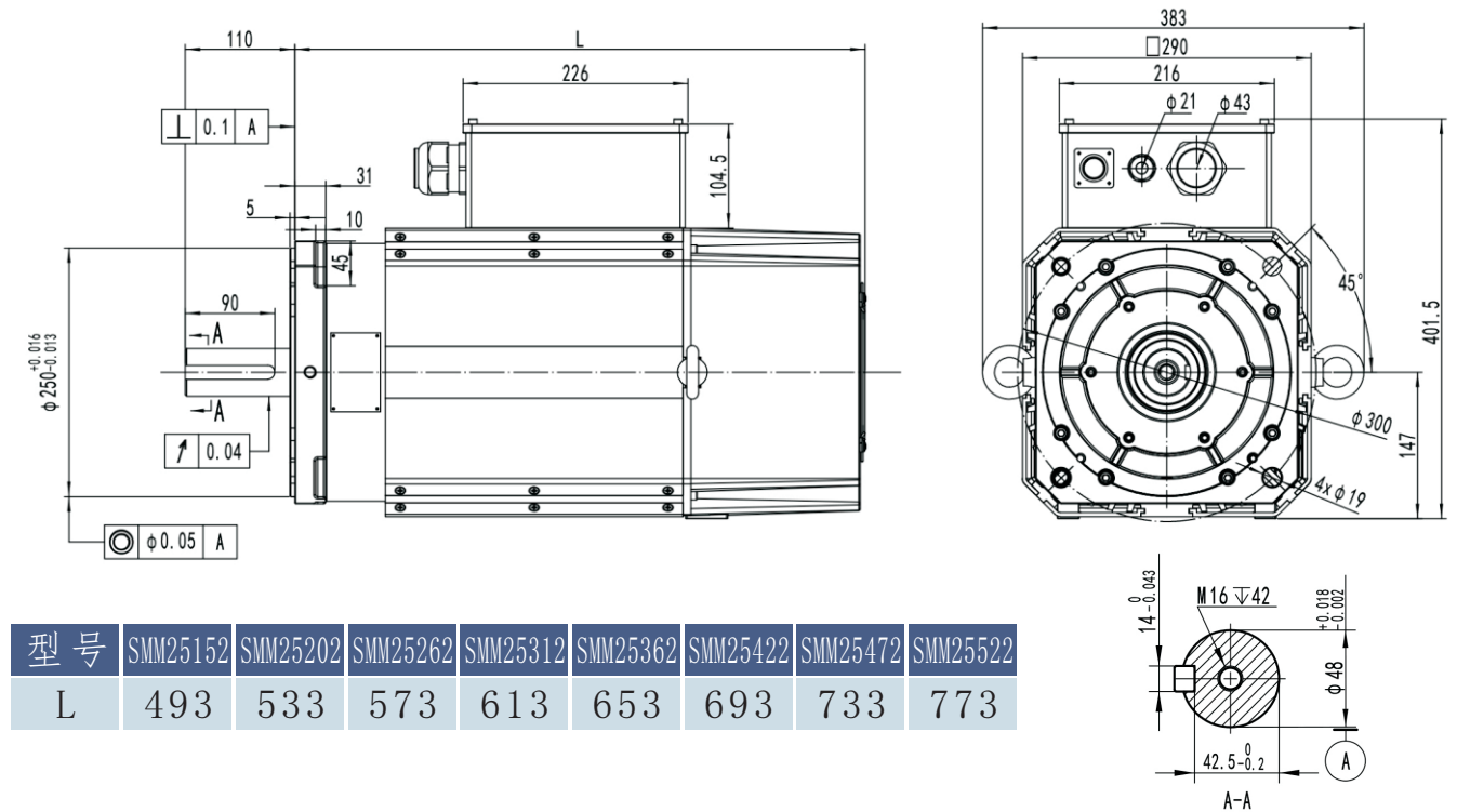
SMM250系列风冷立式电机外形尺寸图&性能参数一览表
