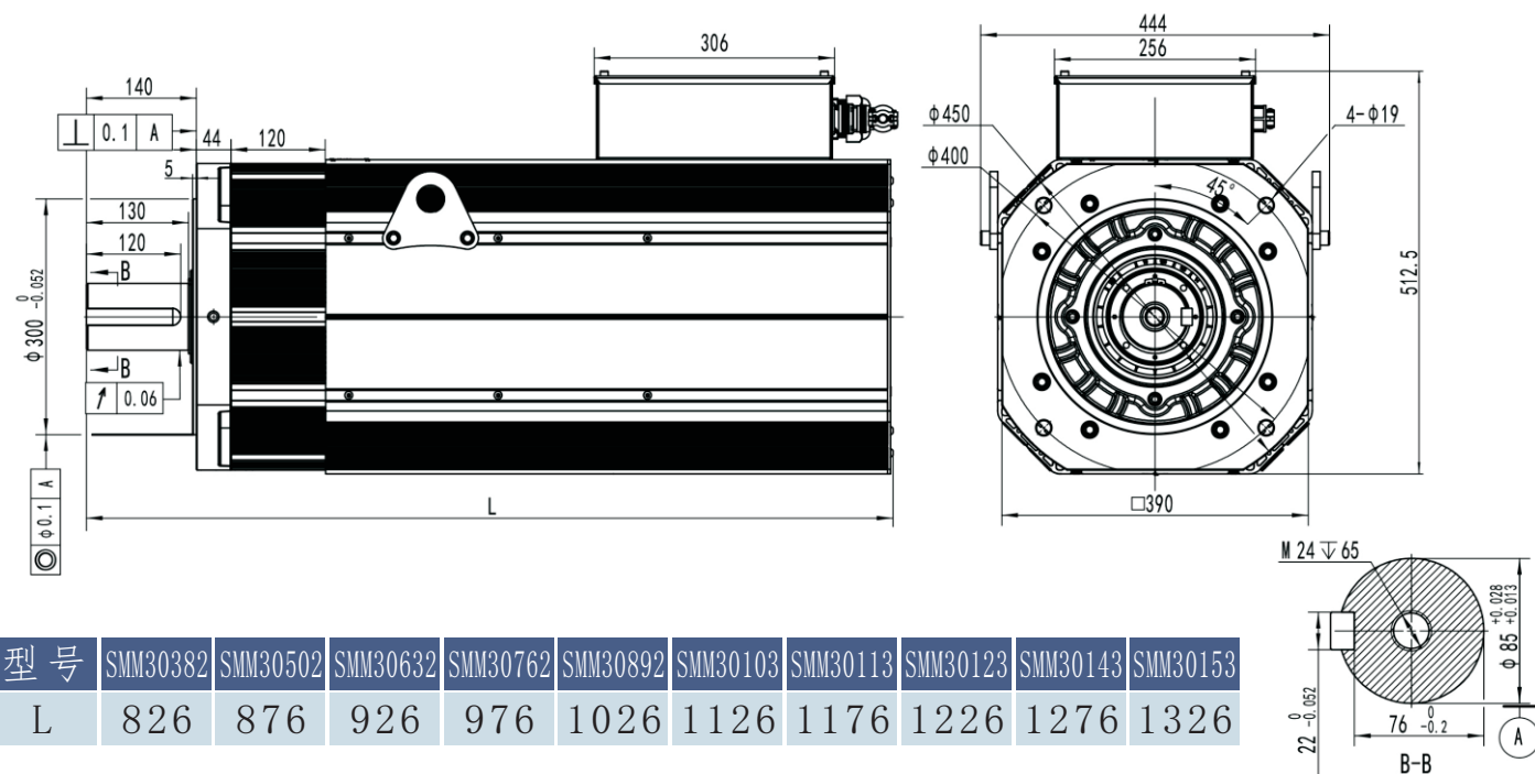
SMM300系列风冷立式电机外形尺寸图&amp;性能参数一览表
