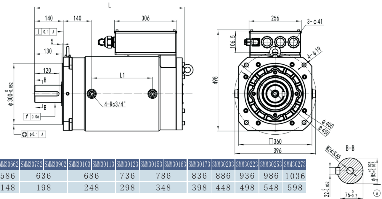
SMM300系列油冷立式熔胶电机外形尺寸图&性能参数一览表
