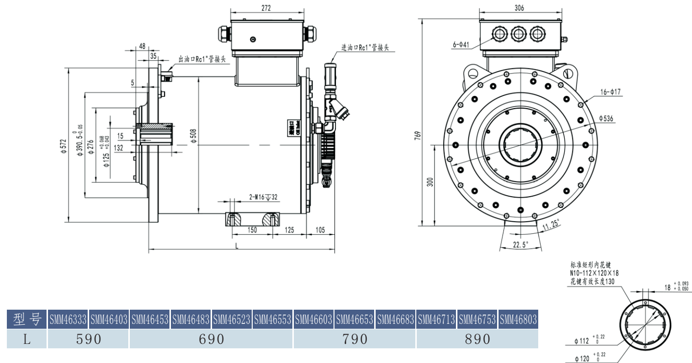
SMM460系列油冷立式熔胶电机外形尺寸图&amp;性能参数一览表
