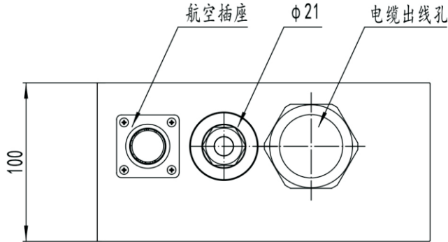
SMM25风冷接线图
