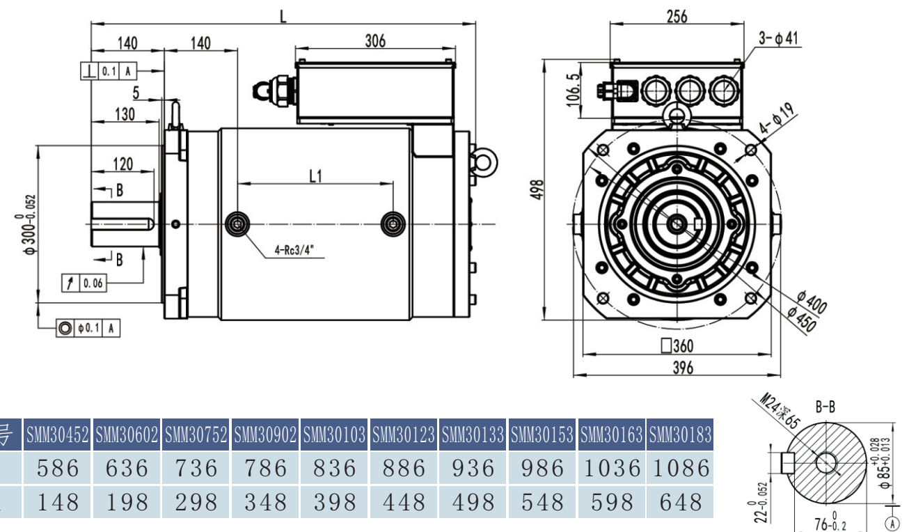
SMM300系列油冷立式电机外形尺寸图&amp;性能参数一览表
