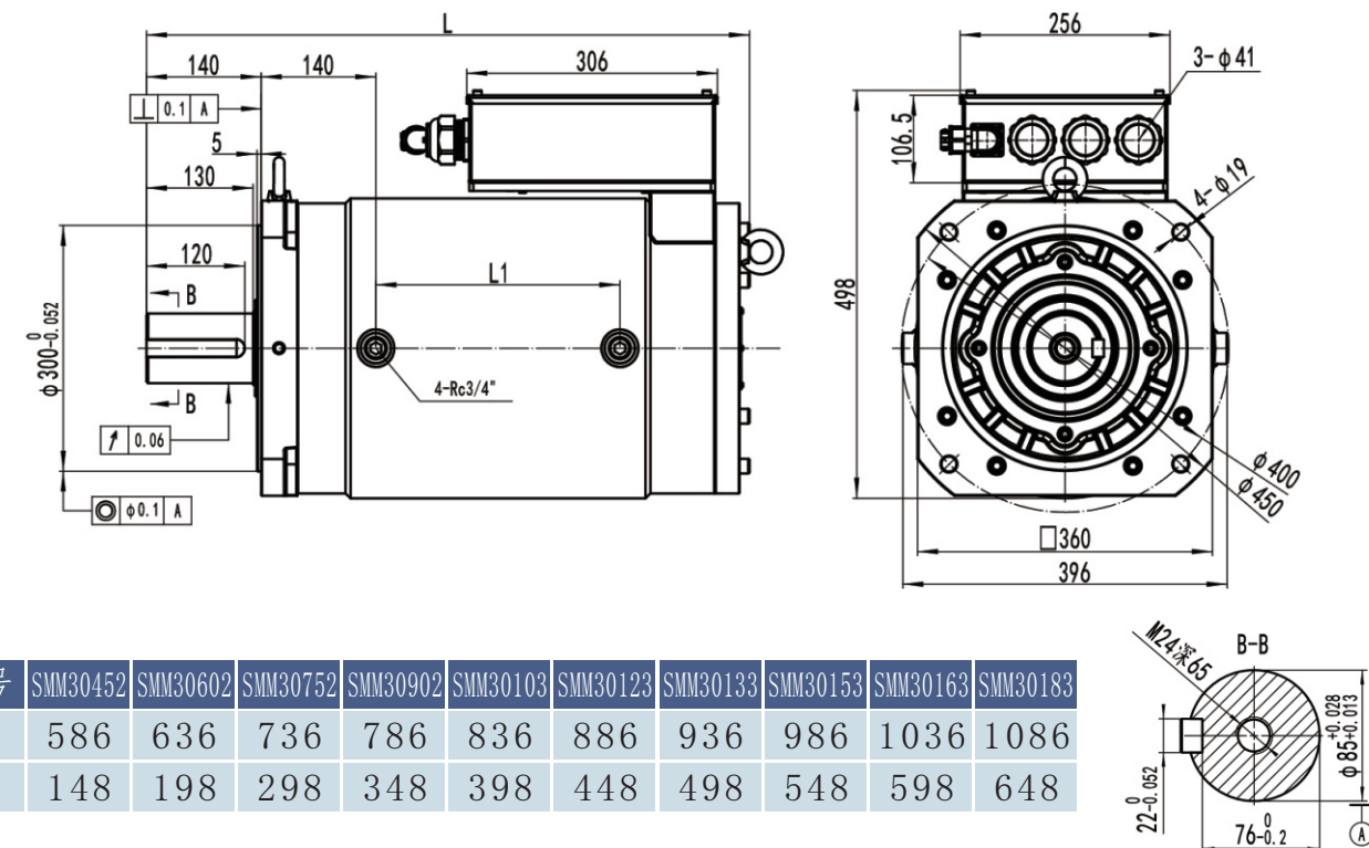
SMM300系列油冷立式熔胶电机外形尺寸图&amp;性能参数一览表
