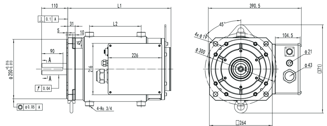
SMM250系列油冷立式电机外形尺寸图&性能参数一览表
