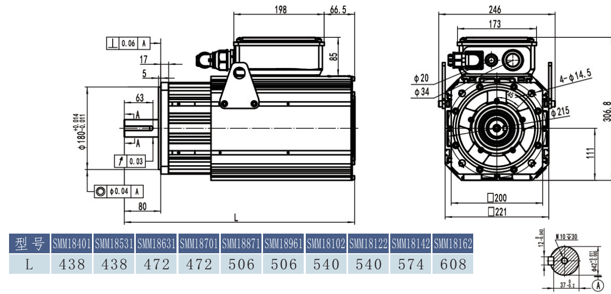
SMM180-H5系列风冷立式电机外形尺寸图&amp;性能参数一览表
