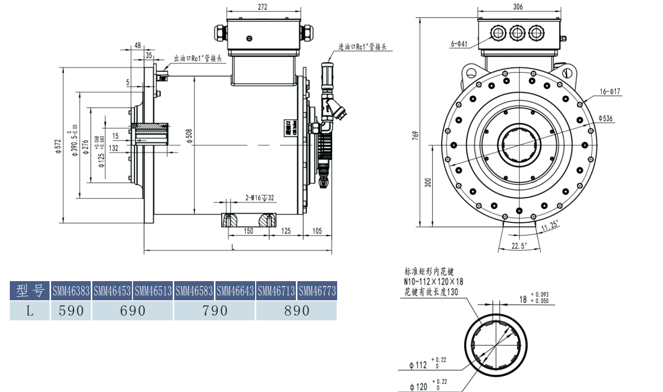
SMM460系列油冷立式熔胶电机外形尺寸图&amp;性能参数一览表
