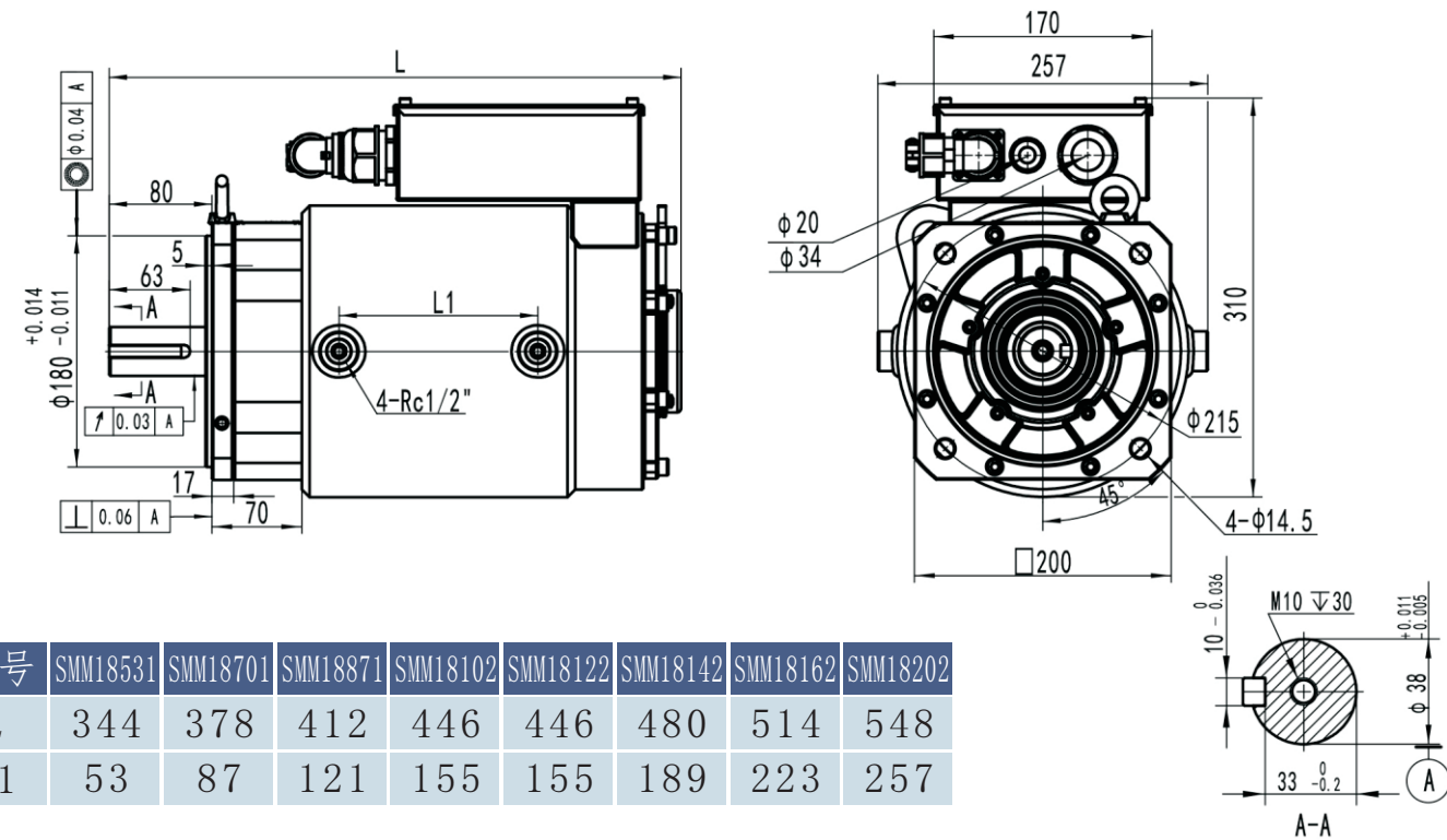
SMM180系列油冷立式电机外形尺寸图&性能参数一览表
